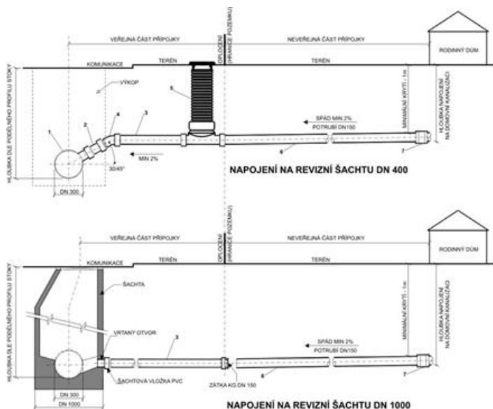
Obrázek vzorového napojení kanalizační přípojky do potrubí kanalizační stoky
